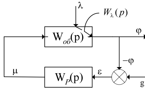
Рис. 2.1. Структурна схема АСК з П-регулятором
