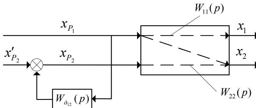
Рис. 4.2 Об'єкт з одним перехресним зв'язком з компенсатором
