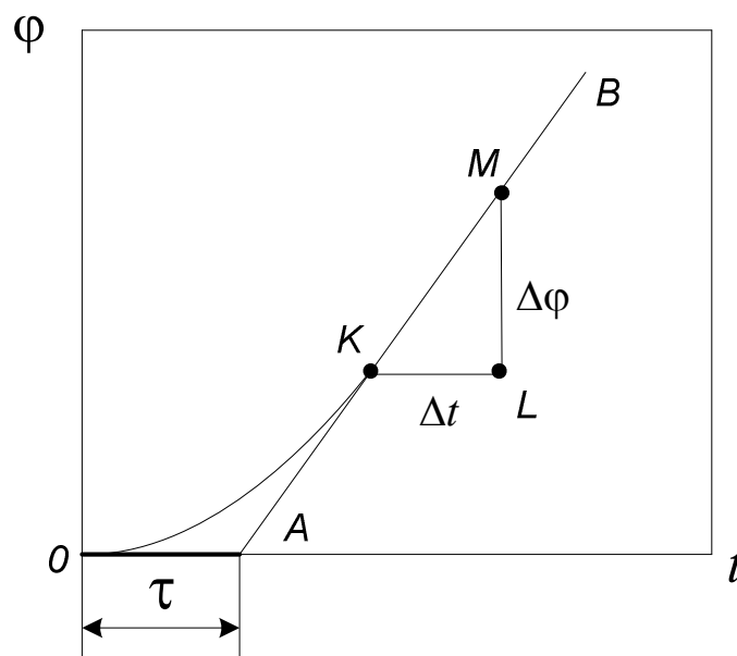
Рис. 5.1 Динамічна характеристика об'єкта без саморегулювання
