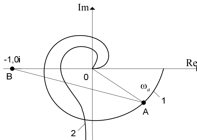
Рис. 3.4 АФХ систем
