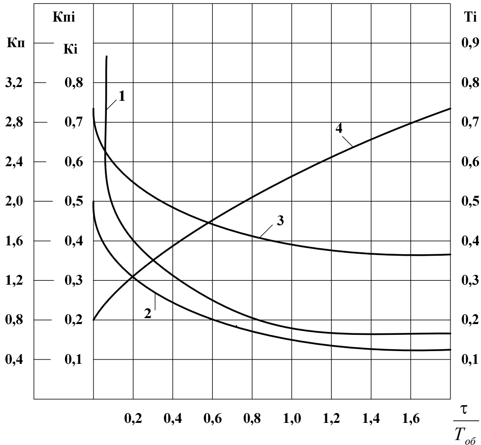
Рис. 5.6 Номограма для визначення параметрів настроювання П-, І-, ІІ-регуляторів 1 – K_{п} ; 2 – K_i ; 3 – K_{пi} ;
